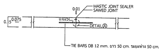
LONGITUDINAL JOINT
