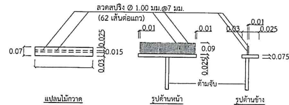
แบบขยายไม่กวาดลาดผิวพื้น ค.ส.ล.
