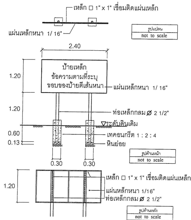
รายละเอียดประกอบแบบ ป้ายชั่วคราวสำหรับโครงการของเทศบาลตำบลท่าไม้รวก
